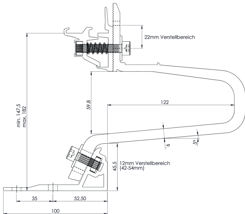
WMS Aludachhaken
